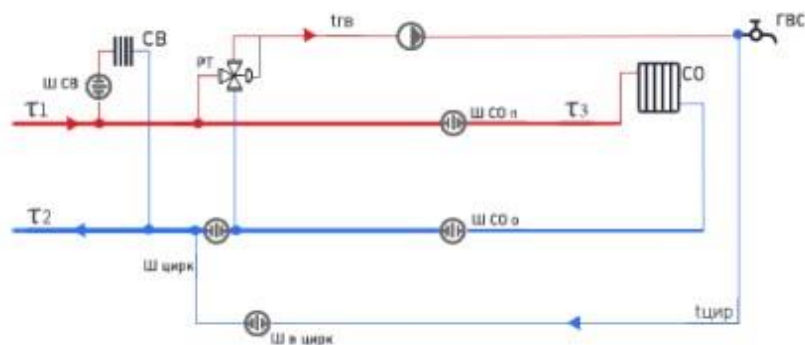
Рисунок 1. Схема присоединения теплотребляющих установок
