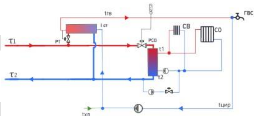
Рисунок 3. Схема присоединения теплотребляющих установок
