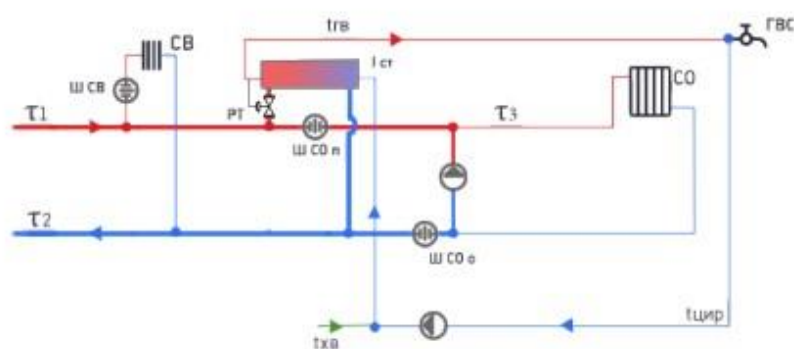
Рисунок 2. Схема присоединения теплотребляющих установок
